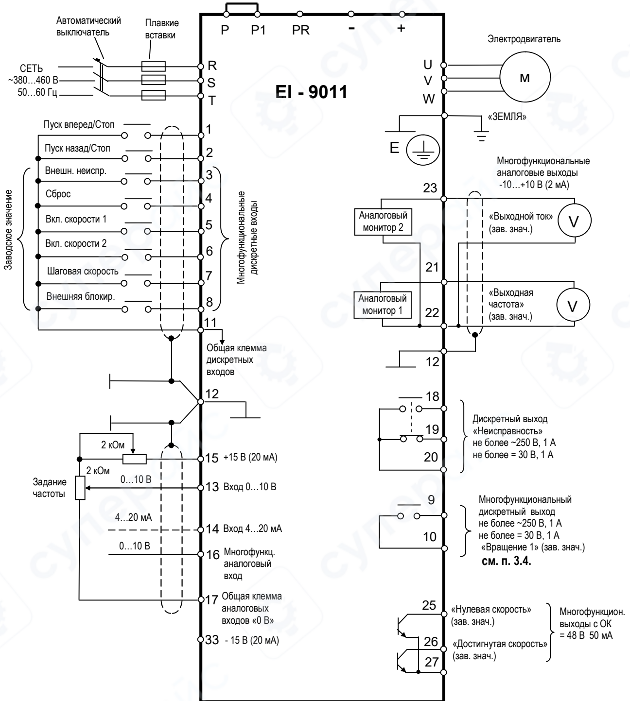
Общая схема подключения EI-9011-001H...600H (020K...600K)
