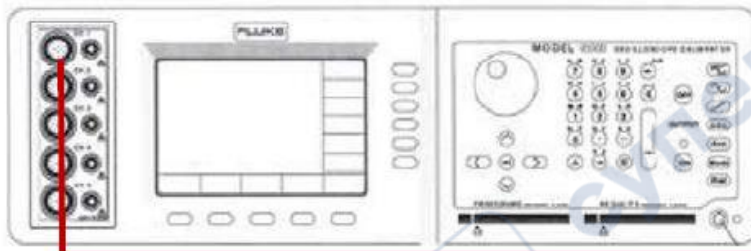
Рисунок 2-5. Схема подключения для испытания точности временной развертки
