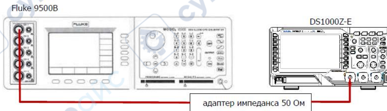
Рисунок 2-6. Схема подключения для испытания смещения нулевой точки
