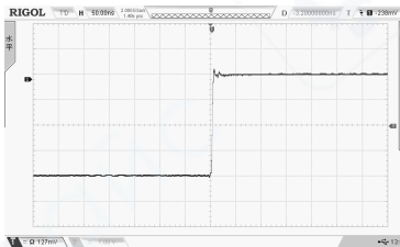
图 3 未添加输入延长线的波形
