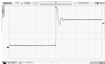
图 4 添加输入延长线（1m）的波形
