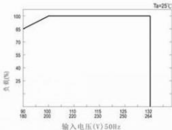
■ 静态特性曲线
