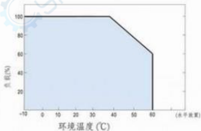
■ 负载减额曲线
