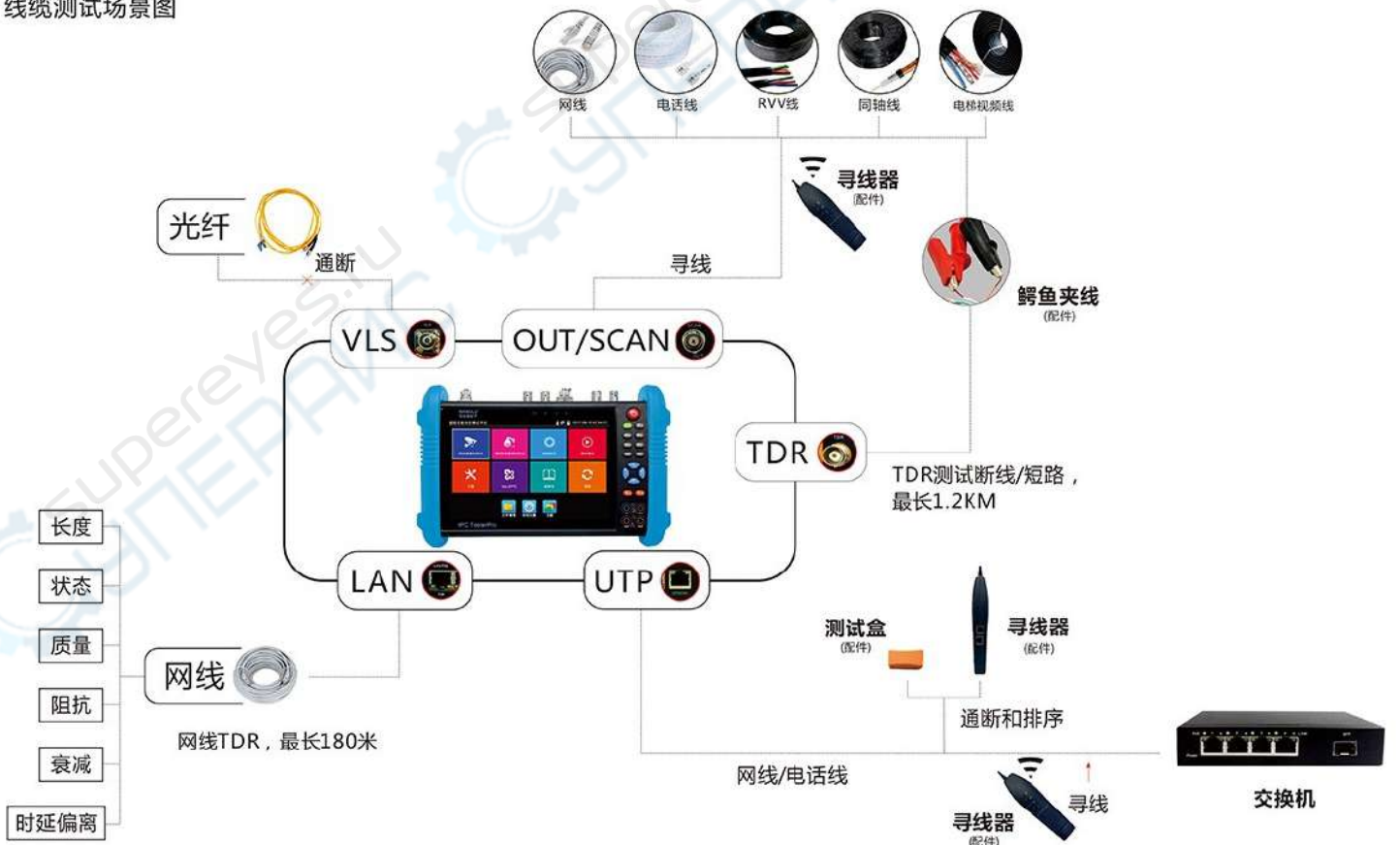
线缆测试场景图
