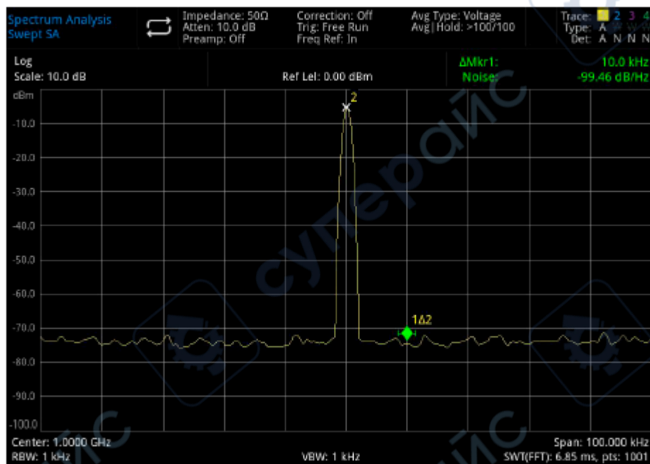
Измерение фазового шума
