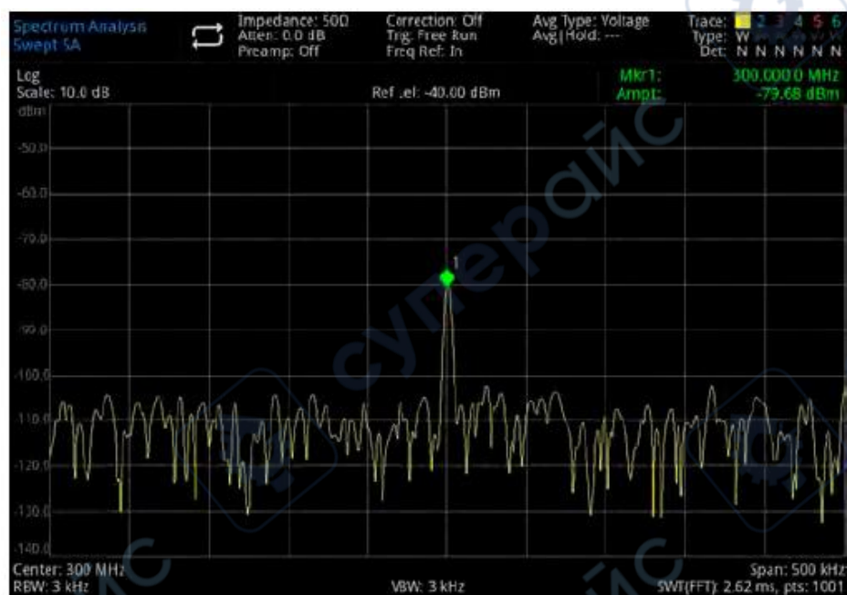
Измерение слабого сигнала при ослаблении 0 дБ
