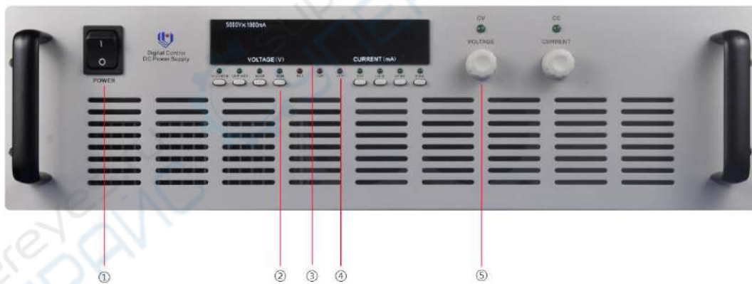
①电源开关 ②功能按键 ③数码显示区域 ④状态指示 ⑤调节区域
