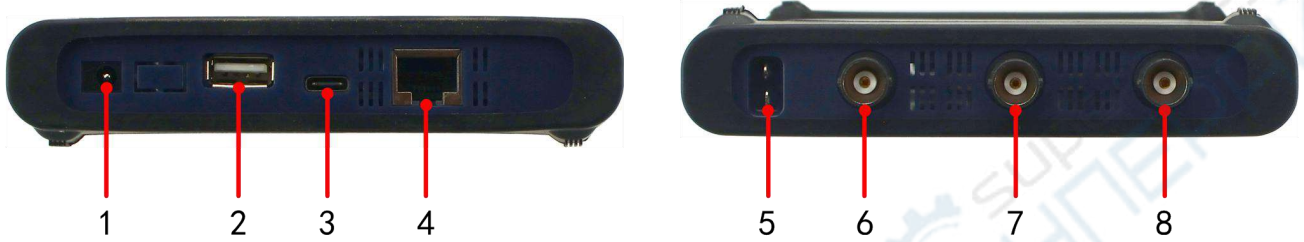
图：示波器接口1
